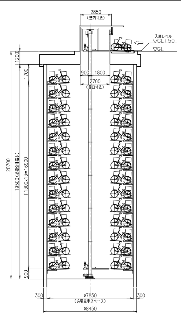
断面図 (側面)
