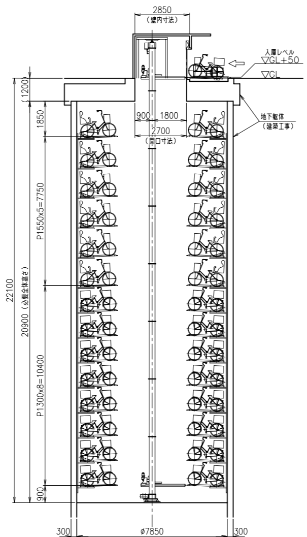
断面図 (側面)
