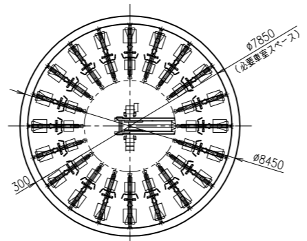
地下平面図
