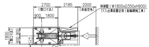
1F平面図
