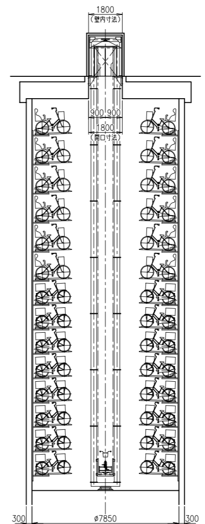
断面図 (正面)
