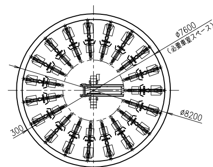
地下平面図
