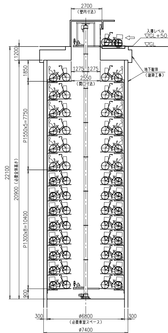
断面図 (側面)
