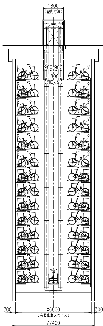
断面図 (正面)
