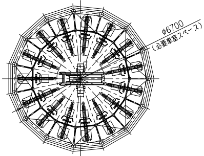
地上平面図
