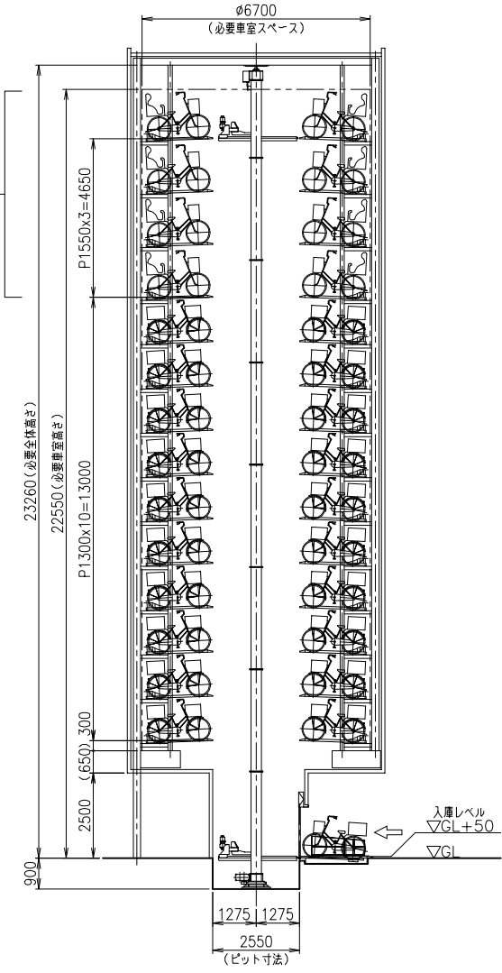
断面図 (側面)
